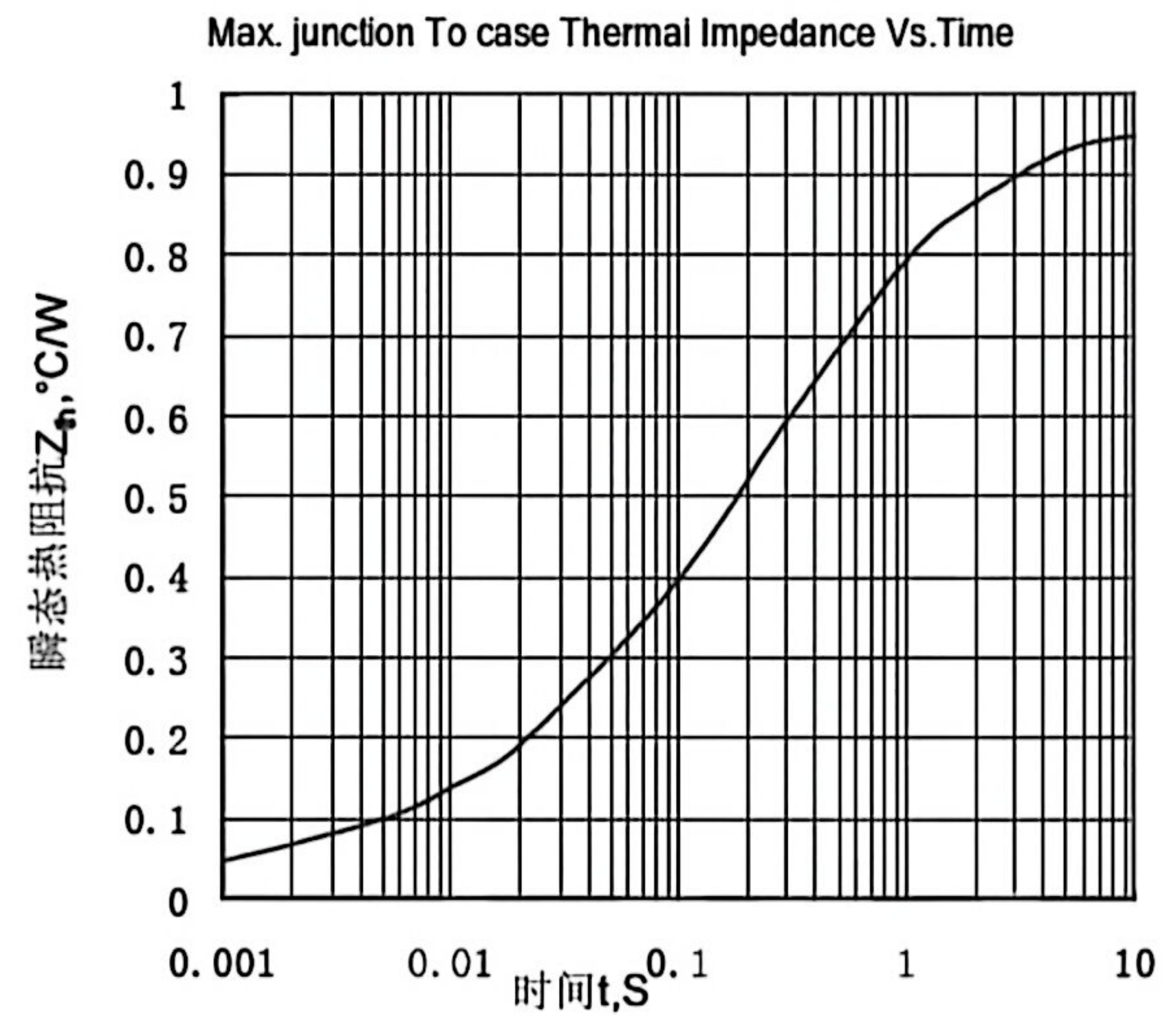
Fig.2 结至管壳瞬态热阻抗曲线
