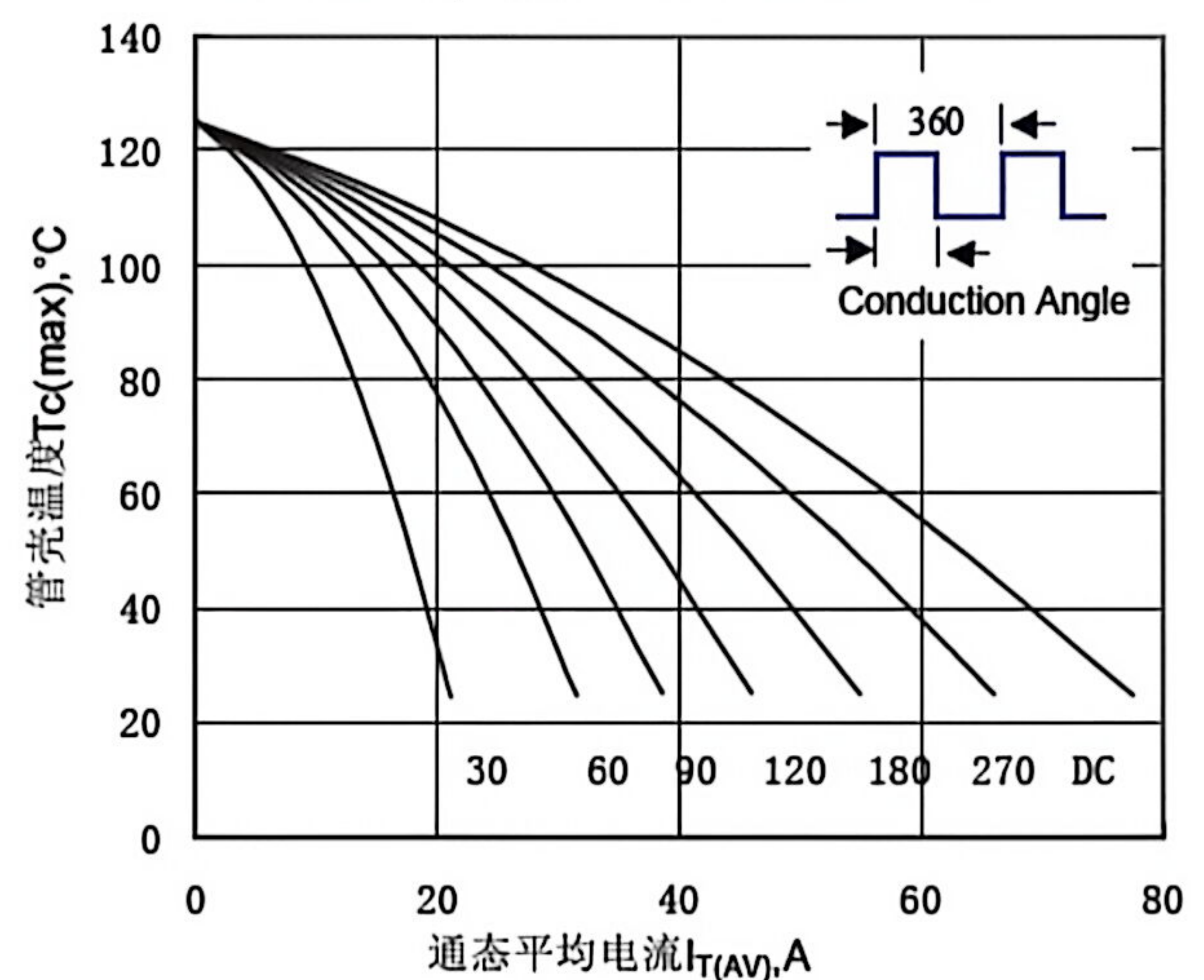
Fig.6 管壳温度与通态平均电流关系曲线
