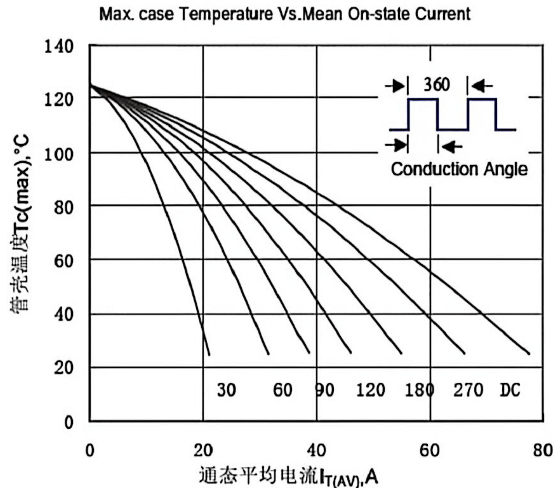
Fig.6 管壳温度与通态平均电流关系曲线
