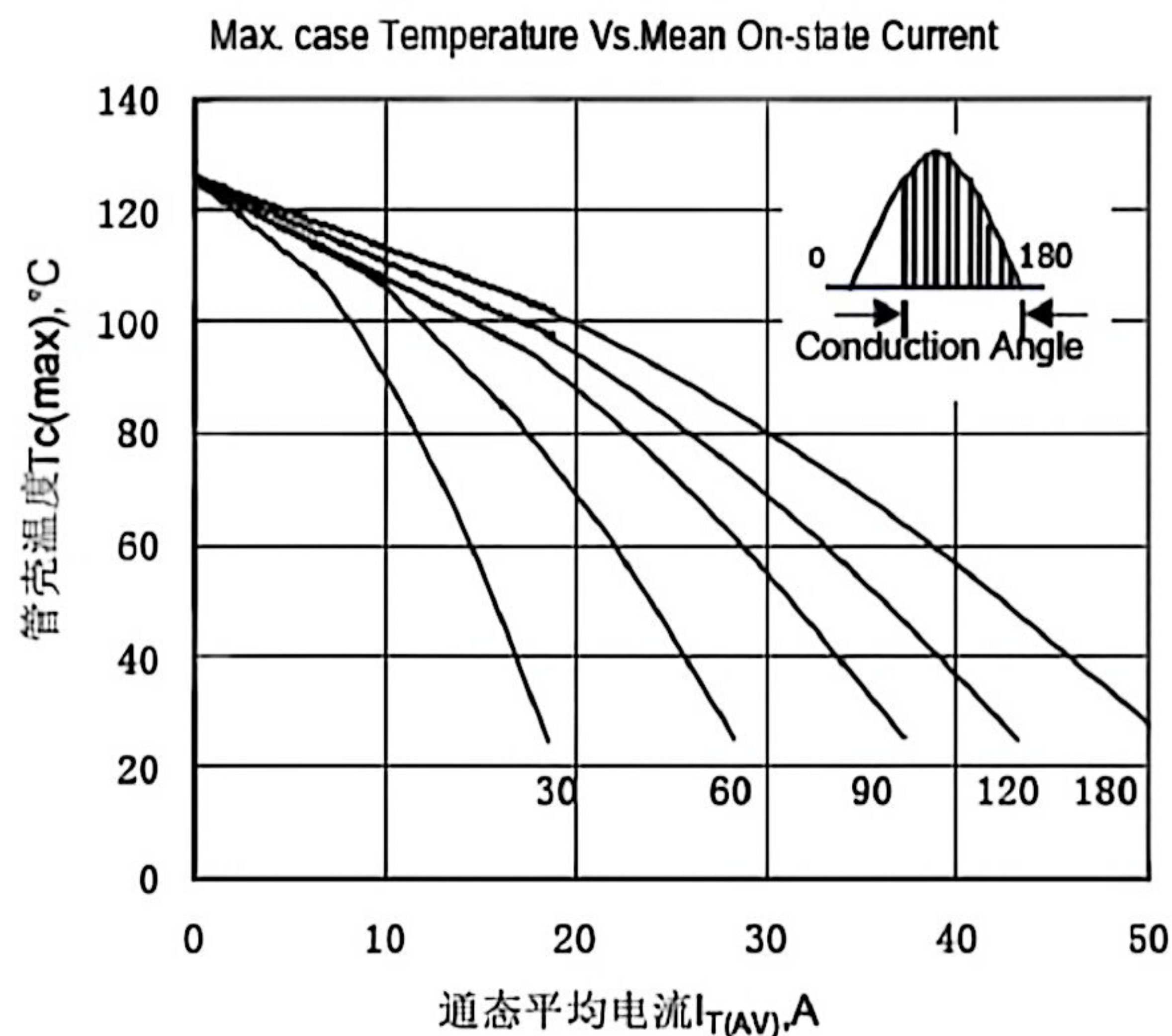
Fig.4 管壳温度与通态平均电流关系曲线
