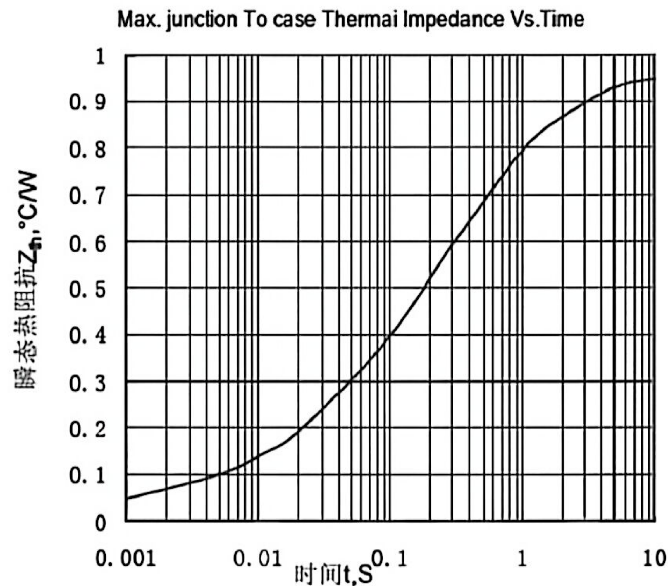
Fig.2 结至管壳瞬态热阻抗曲线
