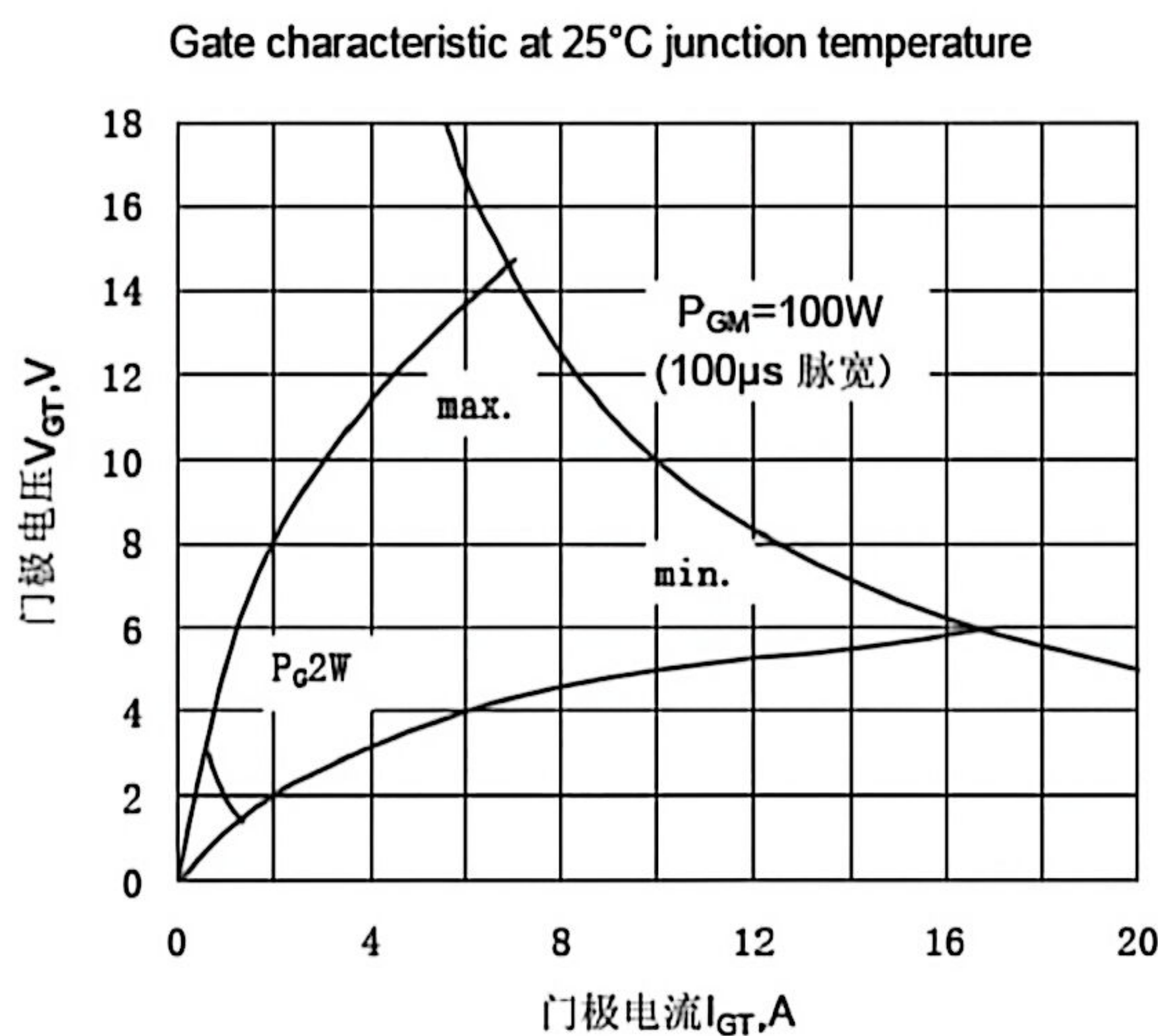
Fig.9 门极功率曲线
