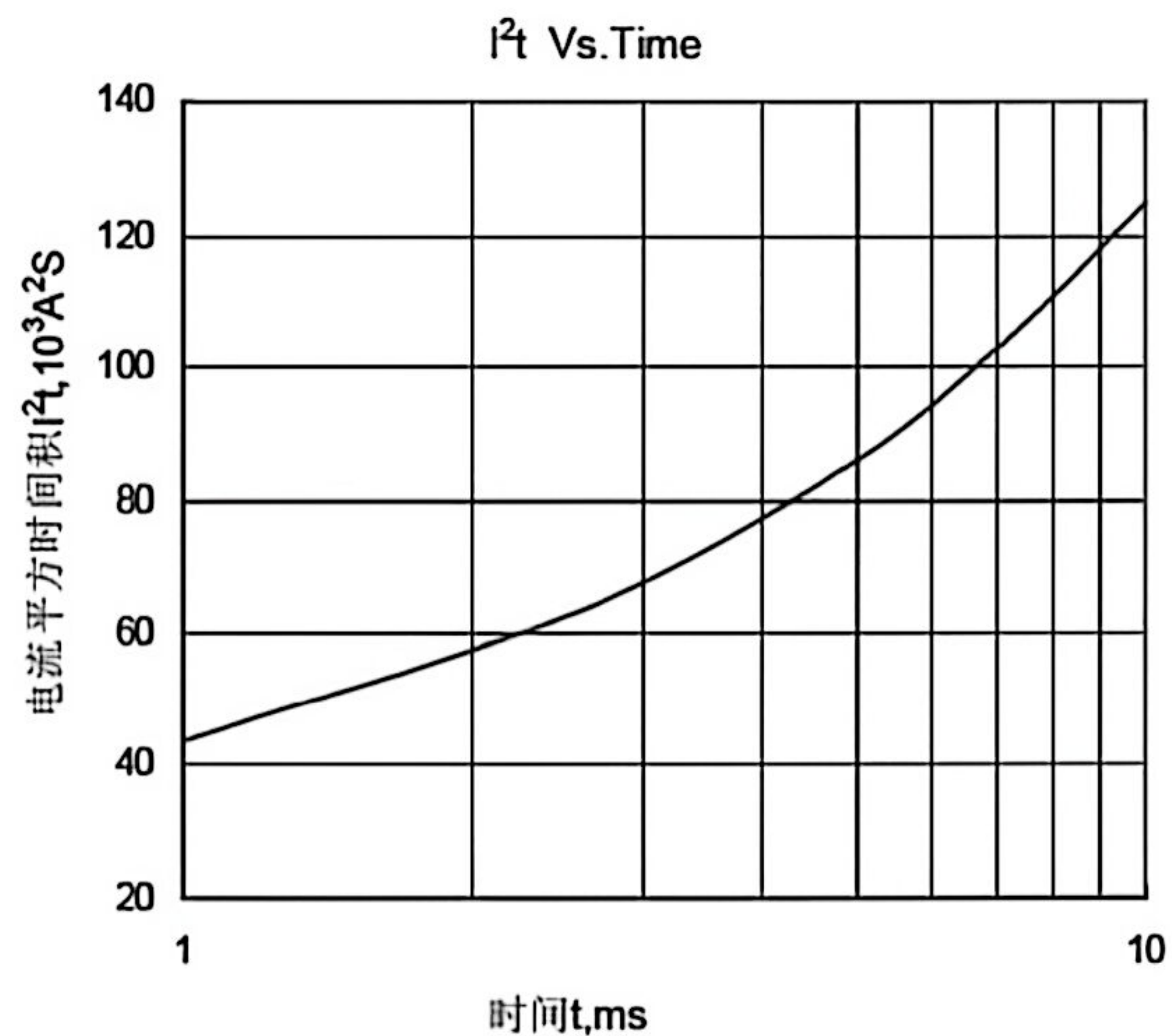
Fig.8 I^2t 特性曲线
