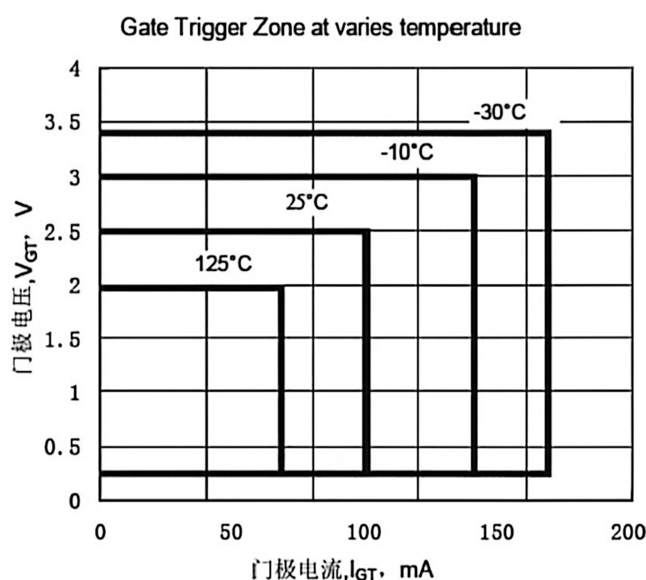
Fig.10 门极触发特性曲线
