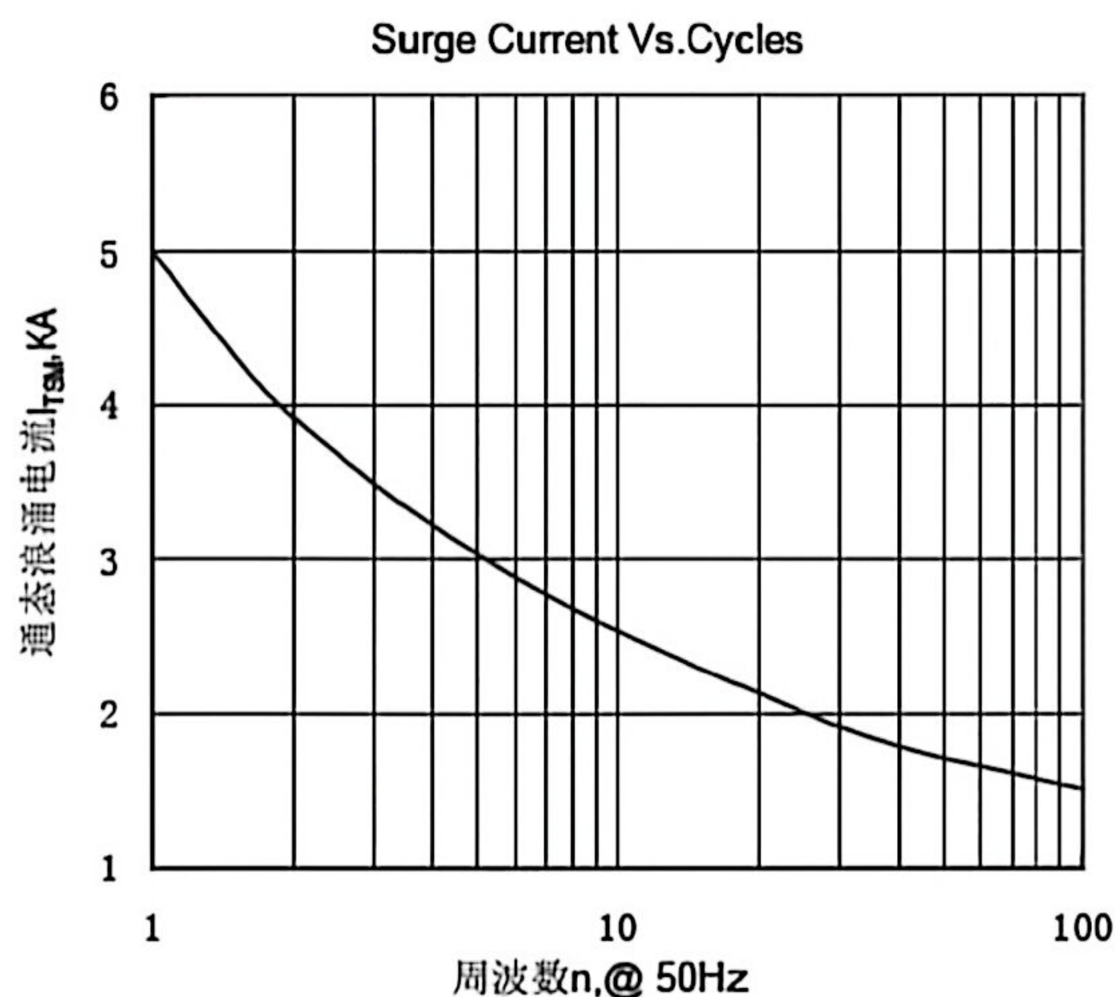
Fig.7 通态浪涌电流与周波数的关系曲线
