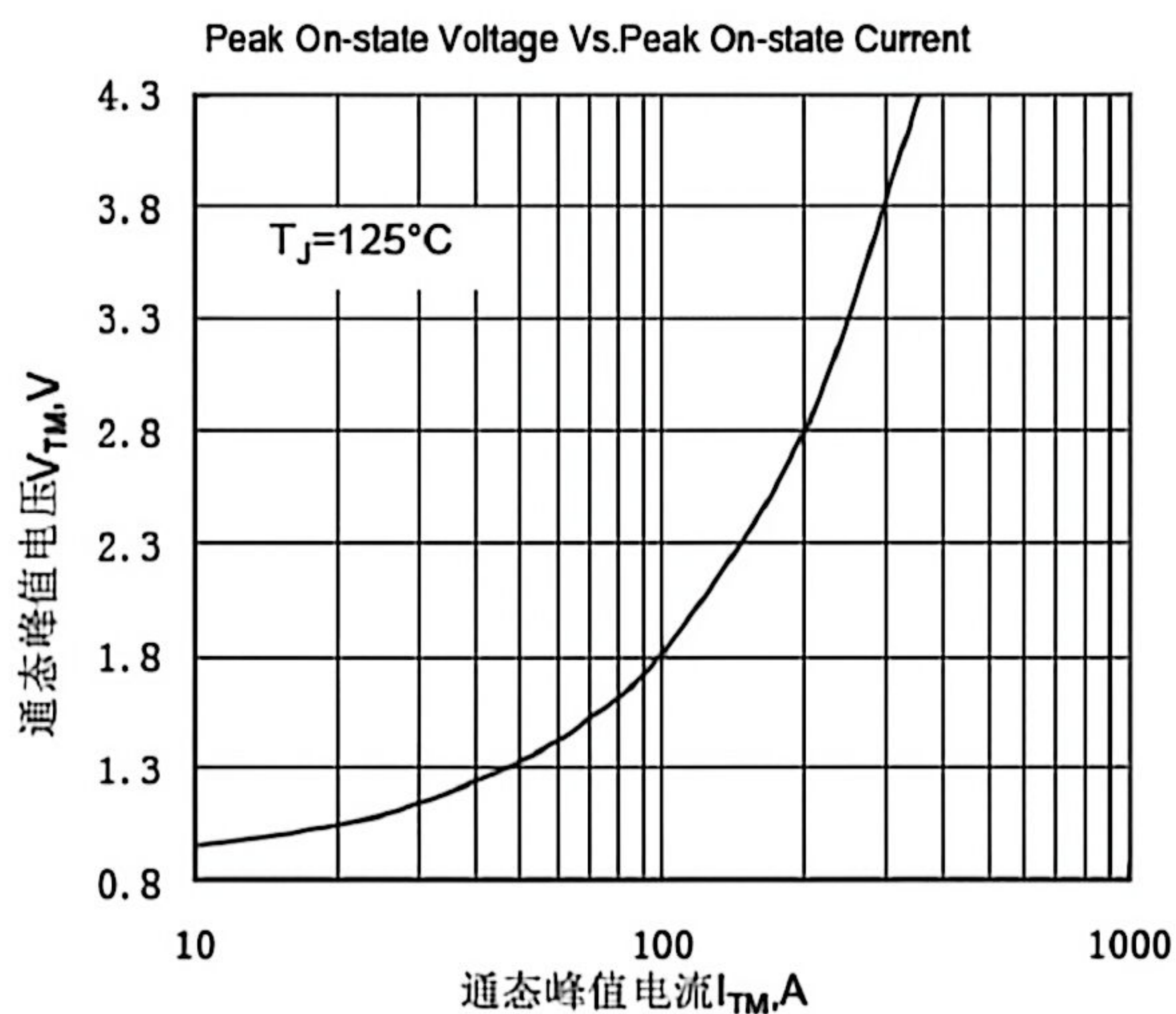
Fig.1 通态伏安特性曲线
