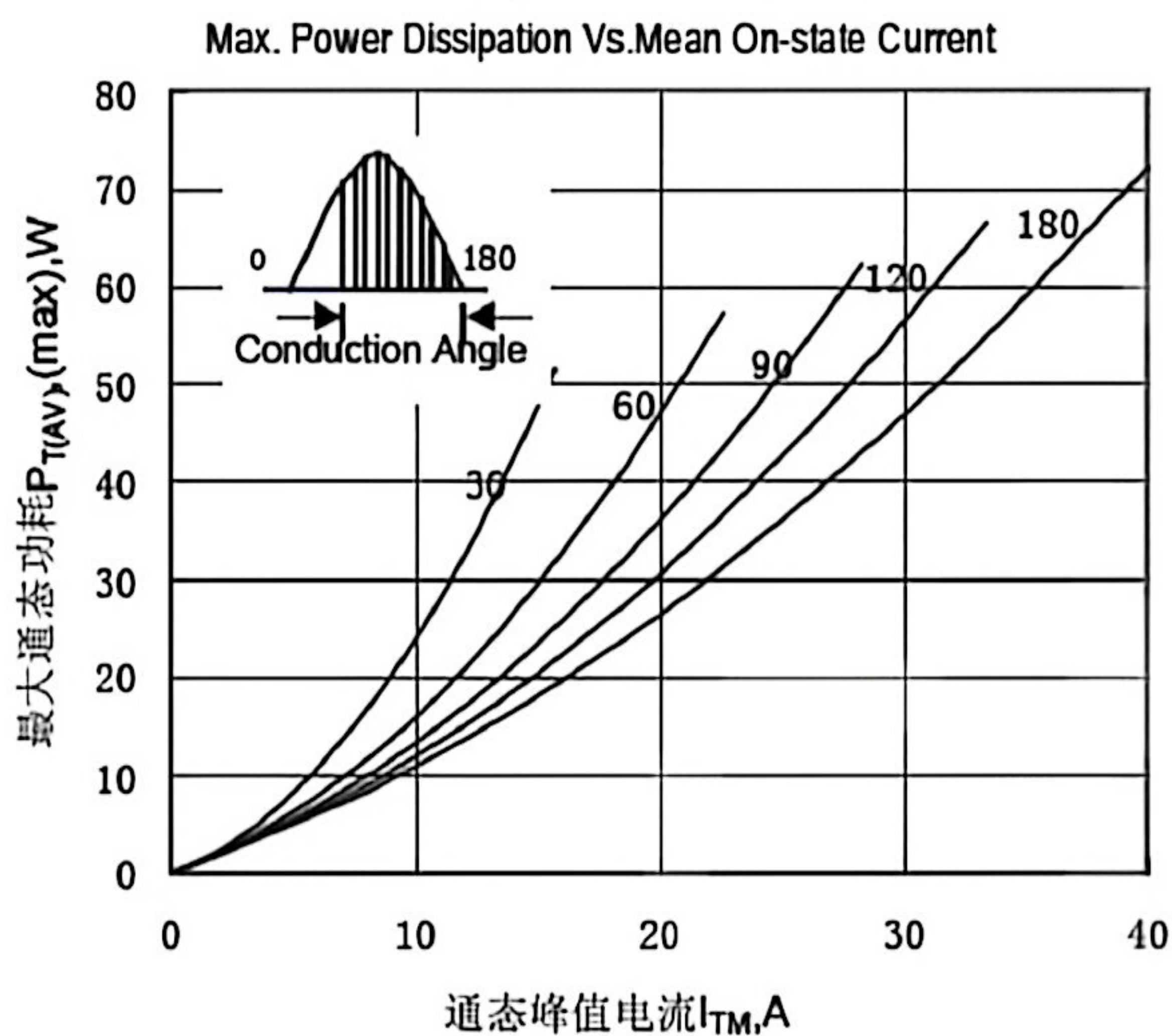
Fig.3 最大功耗与平均电流关系曲线
