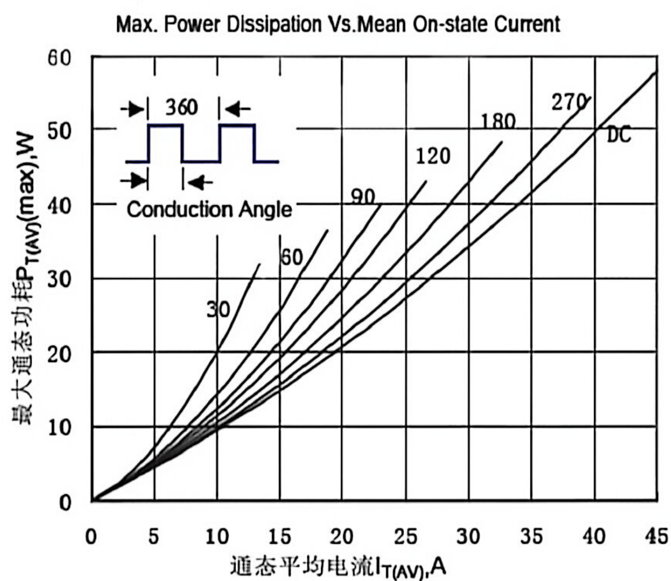
Fig.5 最大功耗与平均电流关系曲线
