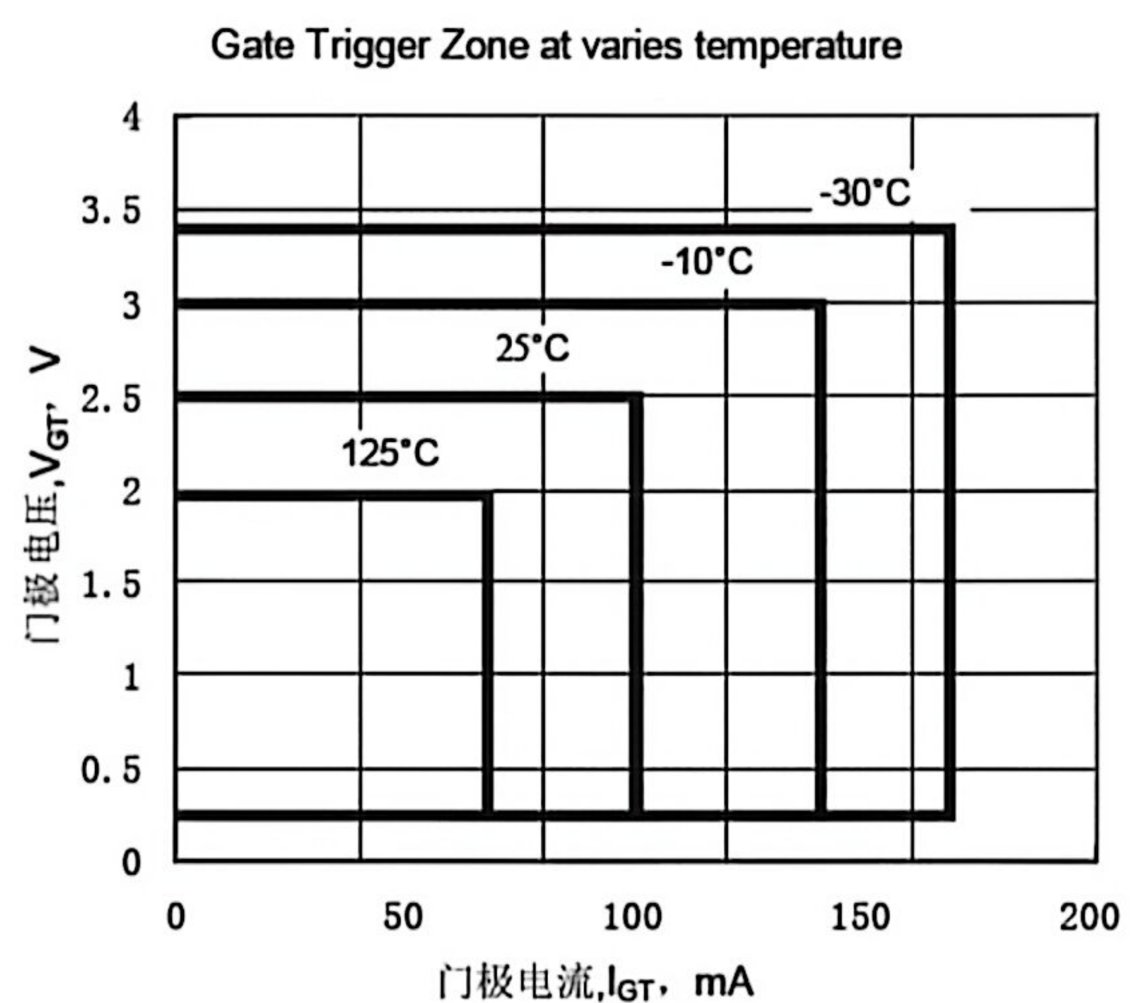
Fig.10 门极触发特性曲线
