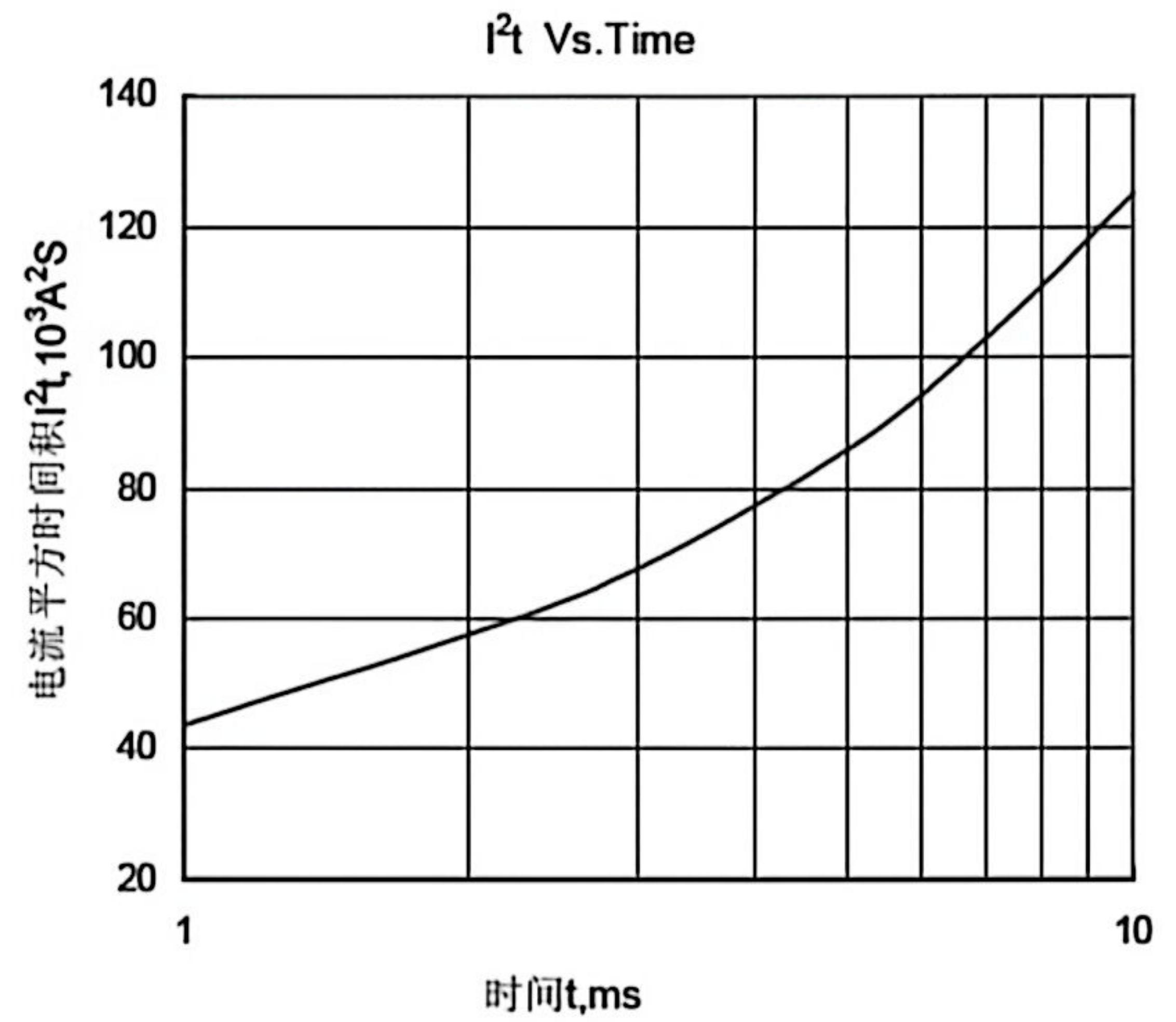
Fig.8 I^2t 特性曲线
