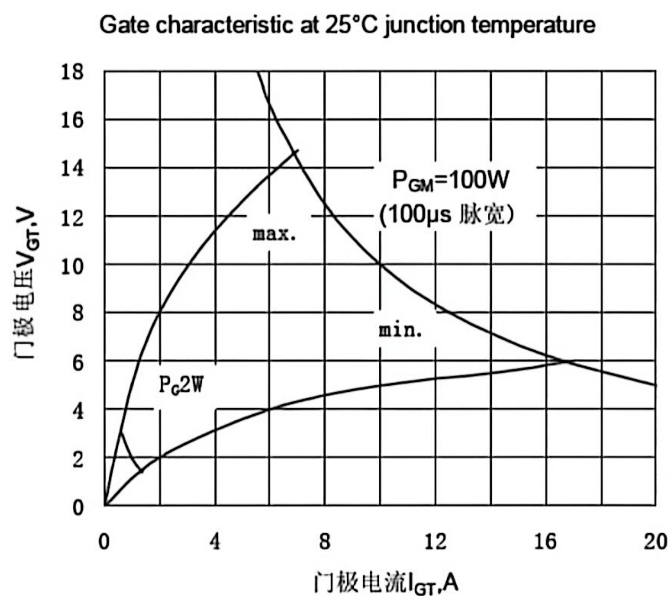
Fig.9 门极功率曲线
