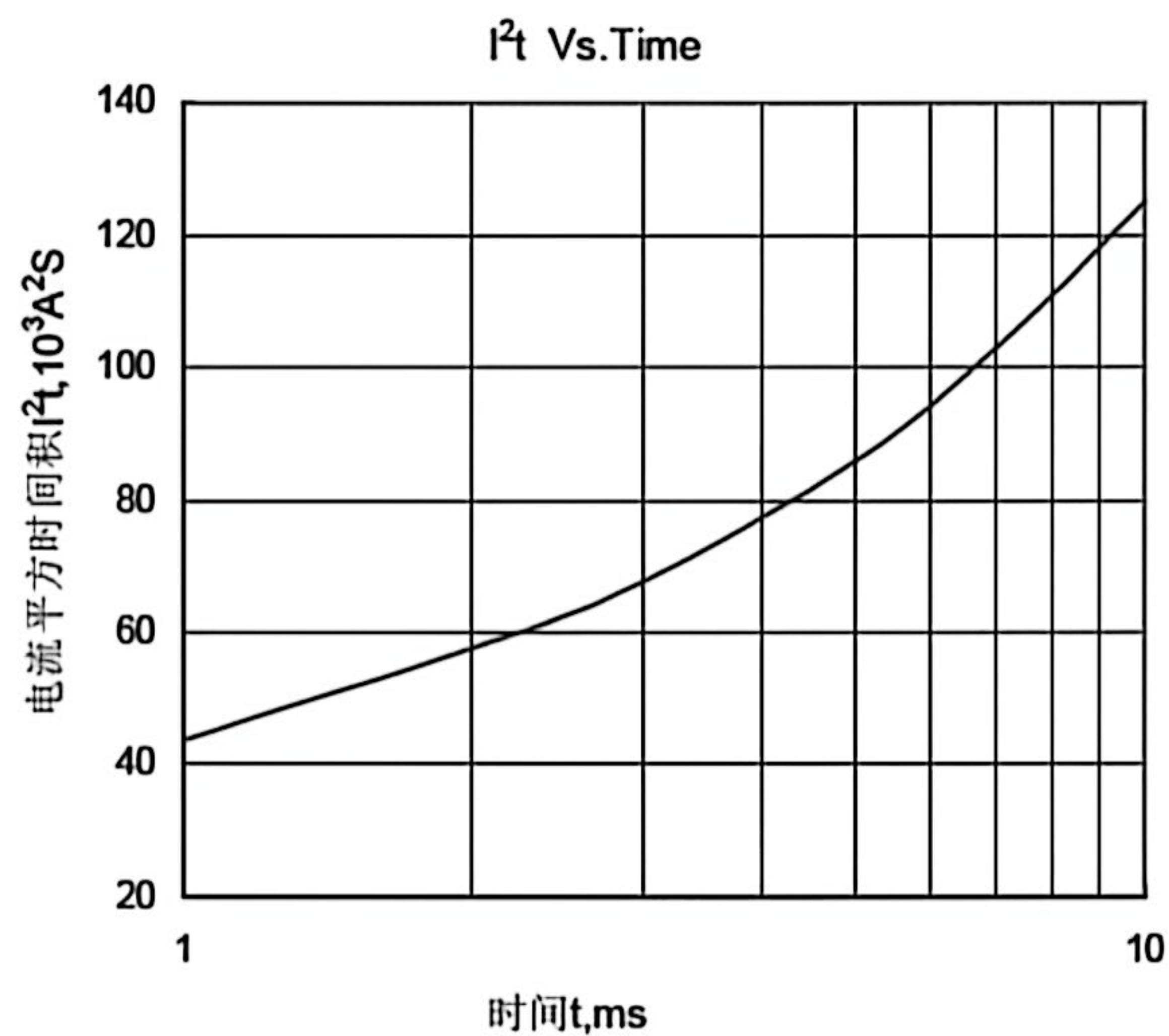
Fig.8 I^2t 特性曲线
