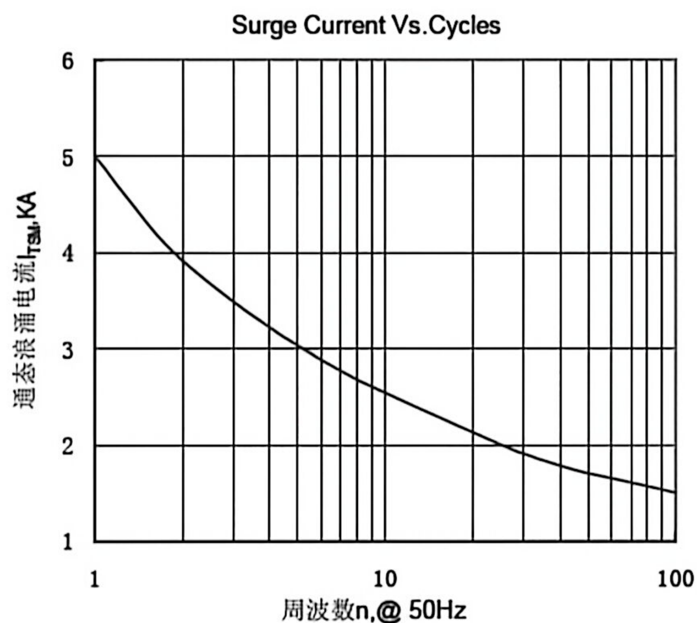
Fig.7 通态浪涌电流与周波数的关系曲线
