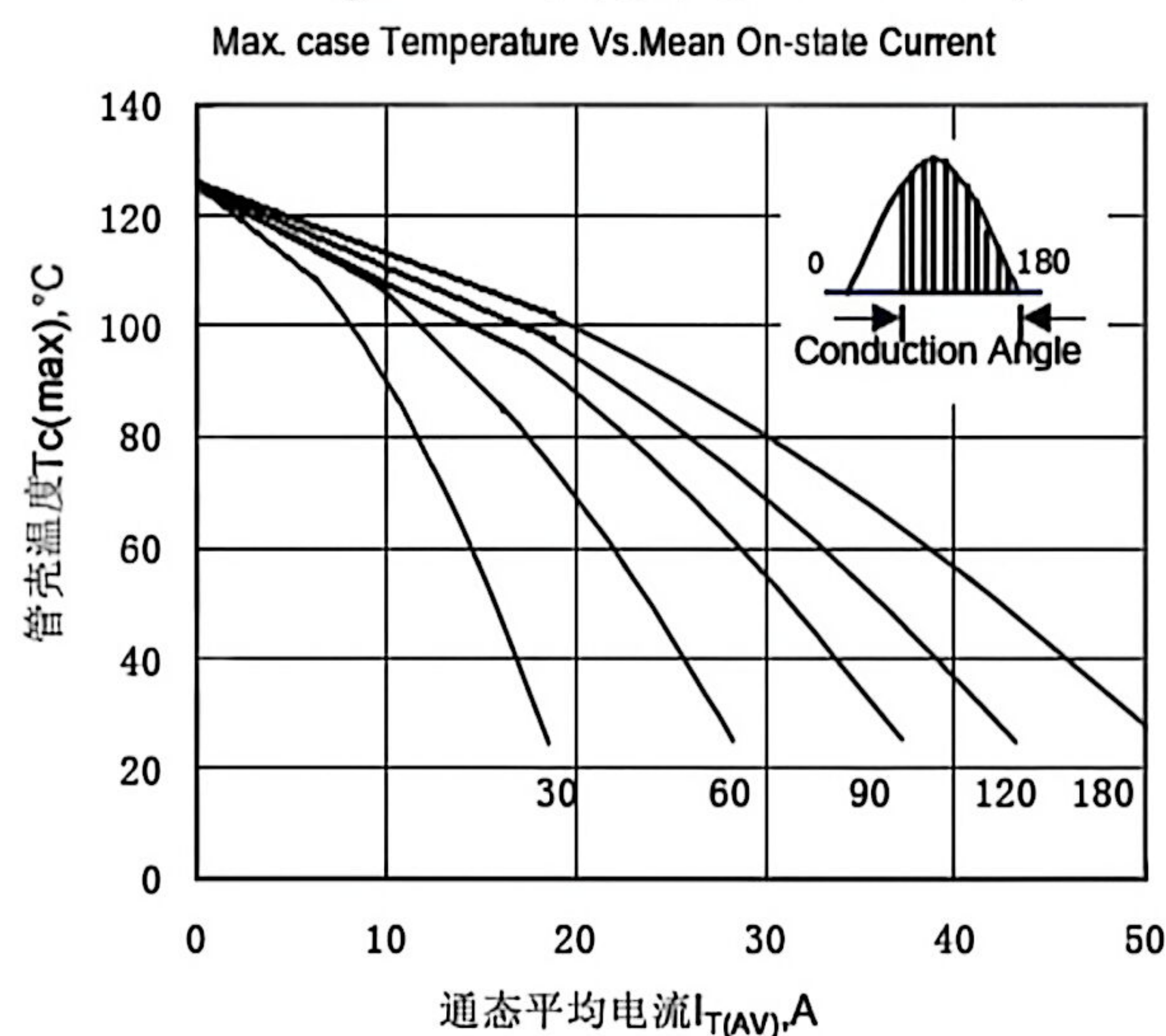
Fig.4 管壳温度与通态平均电流关系曲线
