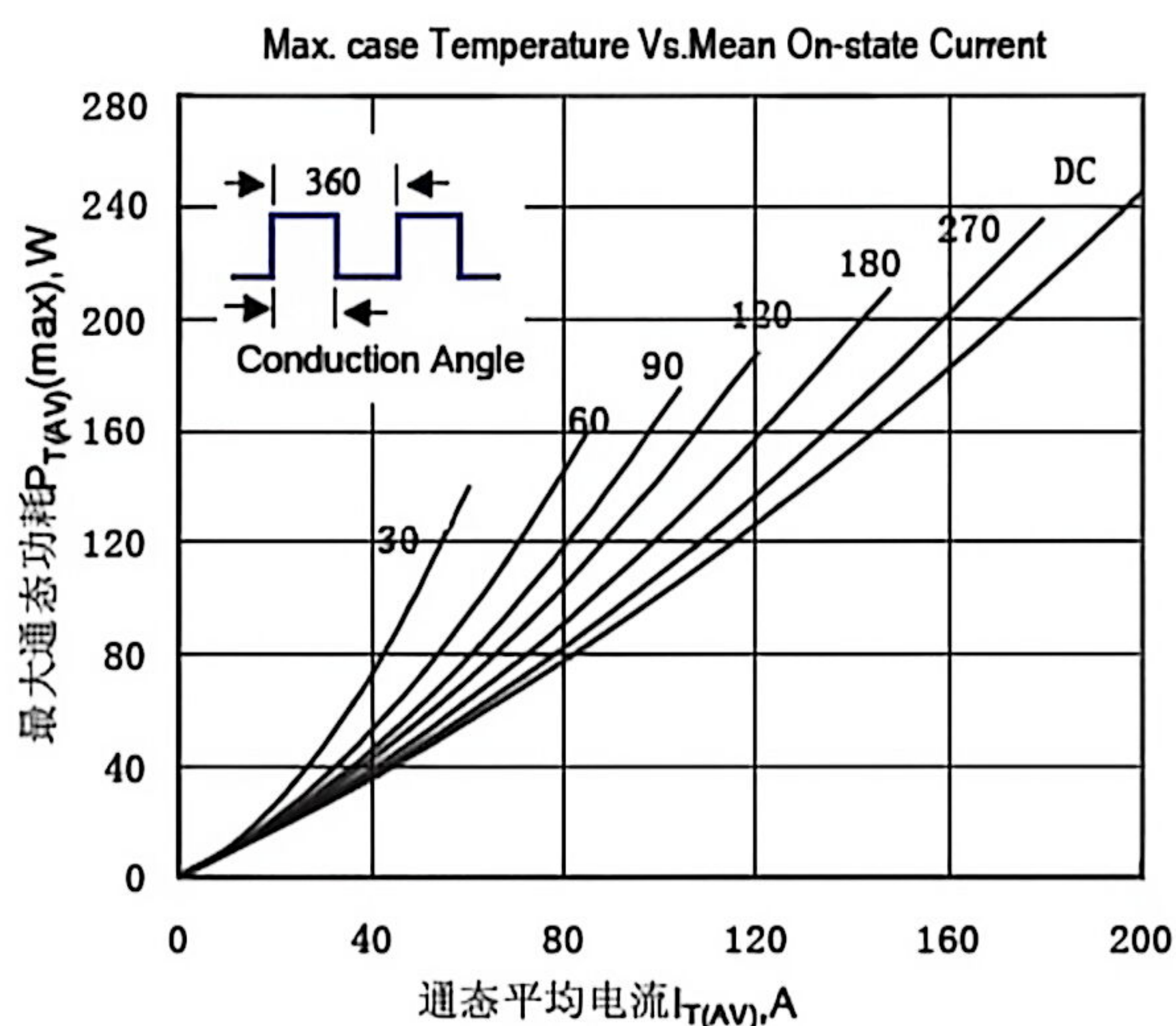
Fig.5 最大功耗与平均电流关系曲线
