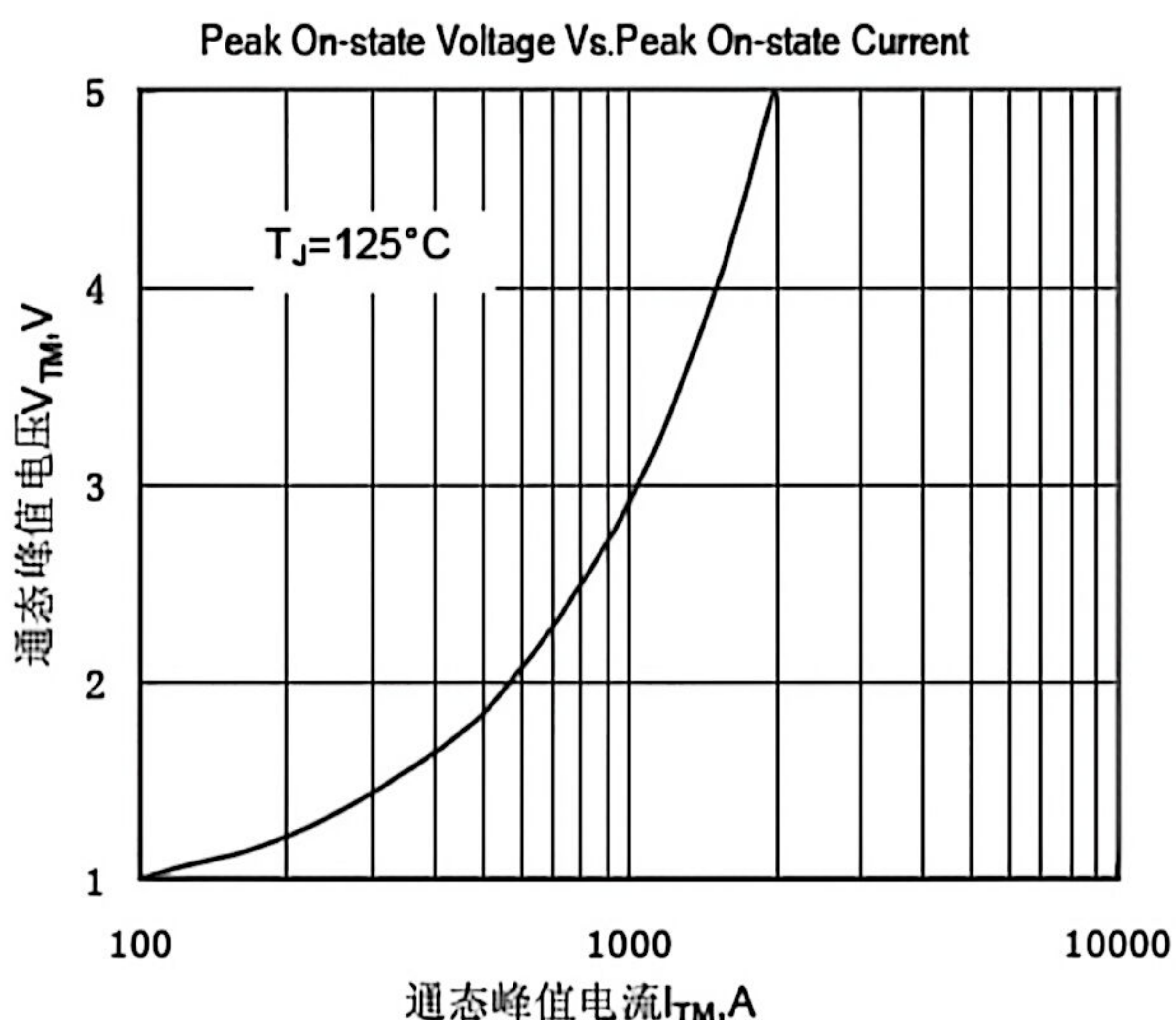
Fig.1 通态伏安特性曲线
